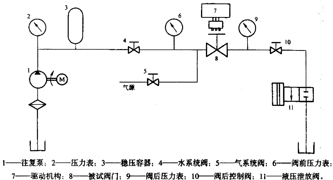
图 1 静压寿命试验系统原理
